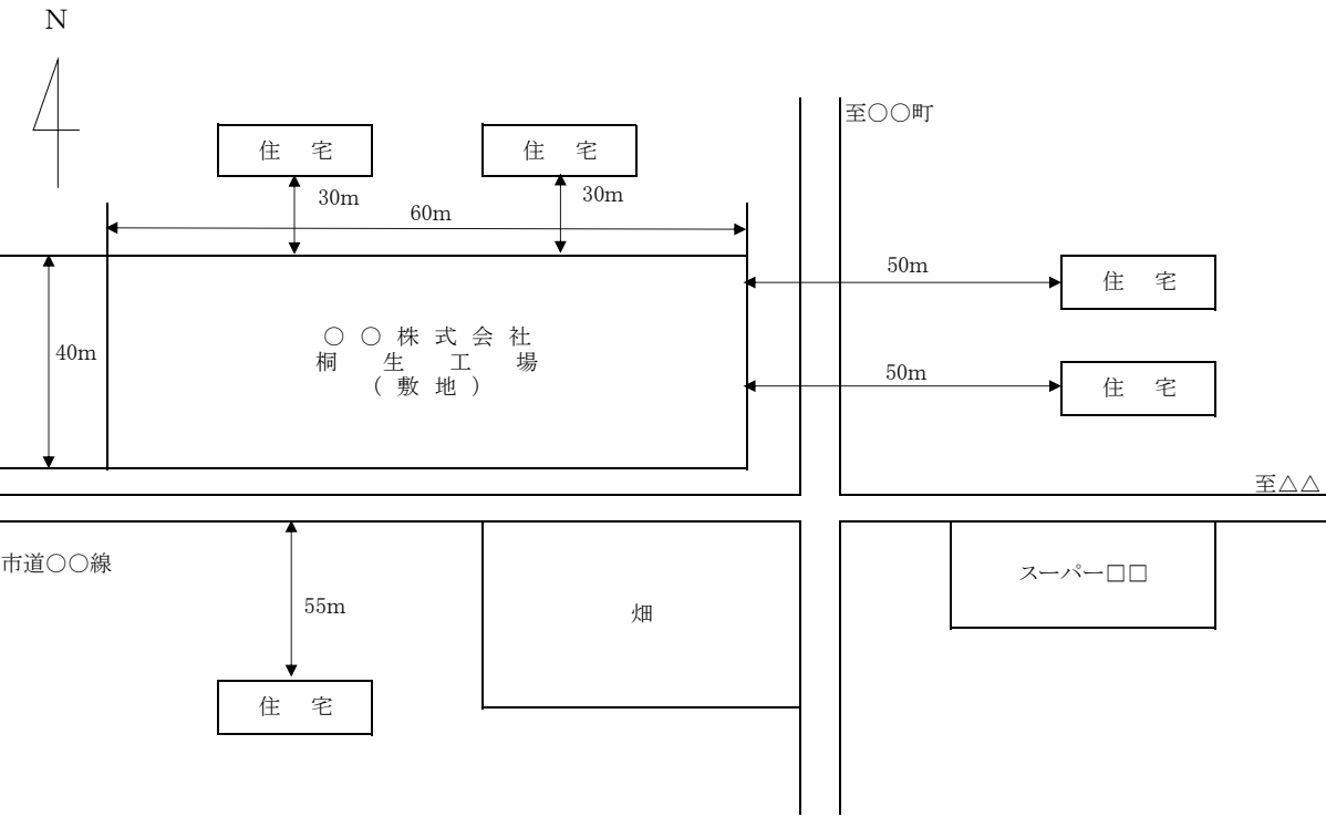
特定工場等の見取図
