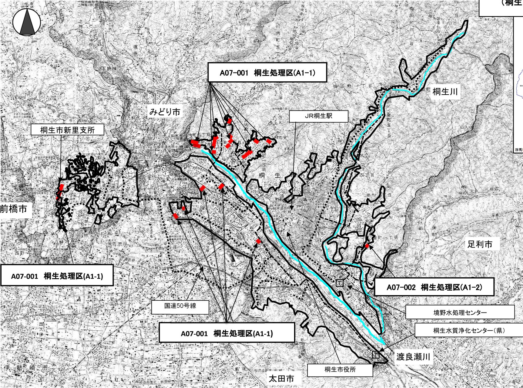
桐生市(A1-1,-2)(桐生処理区、境野処理区)計画図
